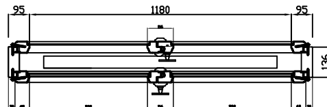
przekrój poziomy pozycja zamknięta
