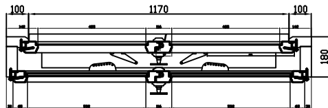
przekrój poziomy pozycja otwarta
